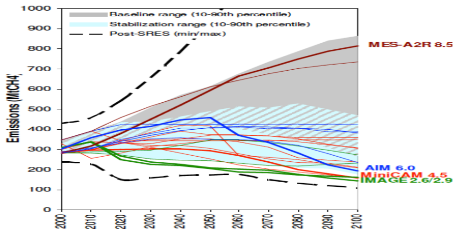
Fig. 4. Evolution des émissions de \text{CH}_4 dans les scénarios du GIEC
