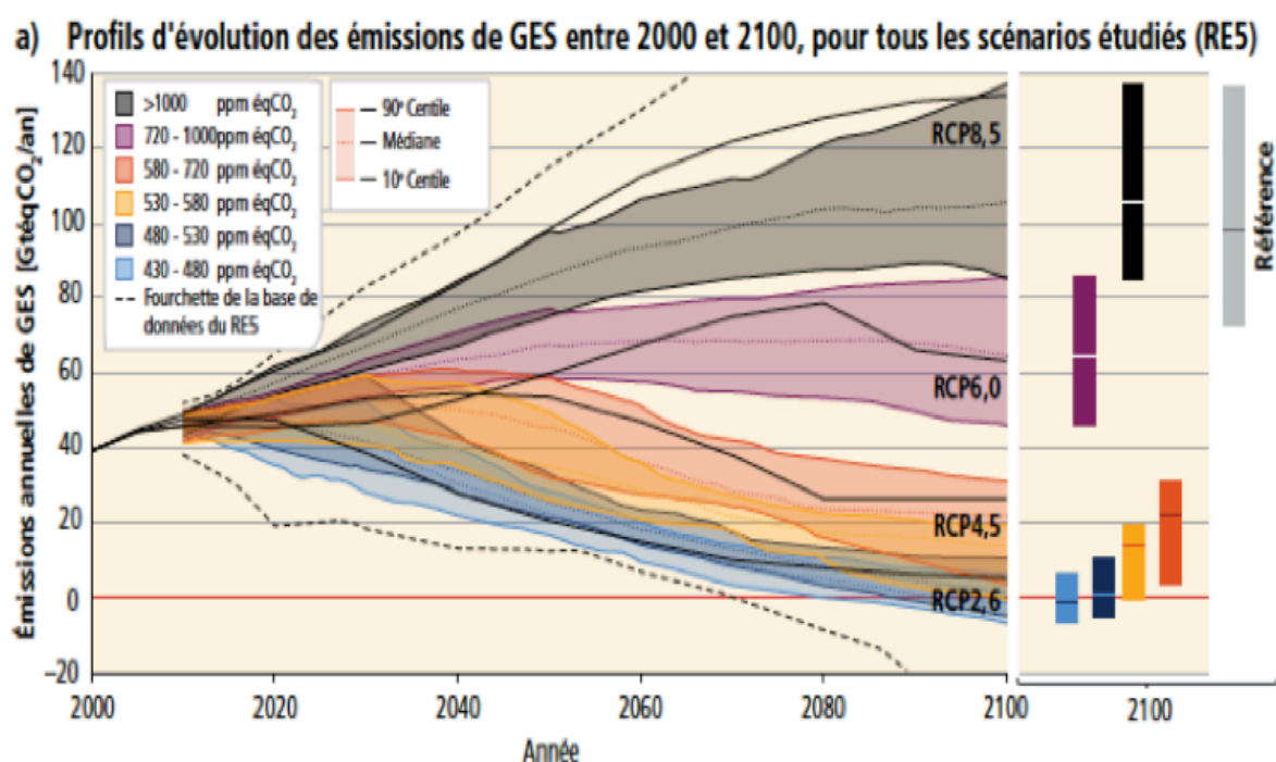
Figure7. Evolution des émissions globales de GES exprimées en \text{GtCO}_2 par an des quatre classes de scénarios de référence du GIEC
