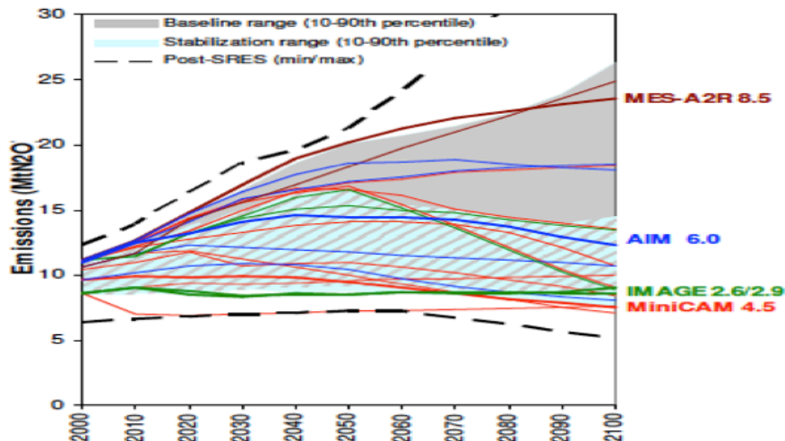
Fig. 5. Evolution des émissions de \text{N}_2\text{O} dans les scénarios du GIEC
