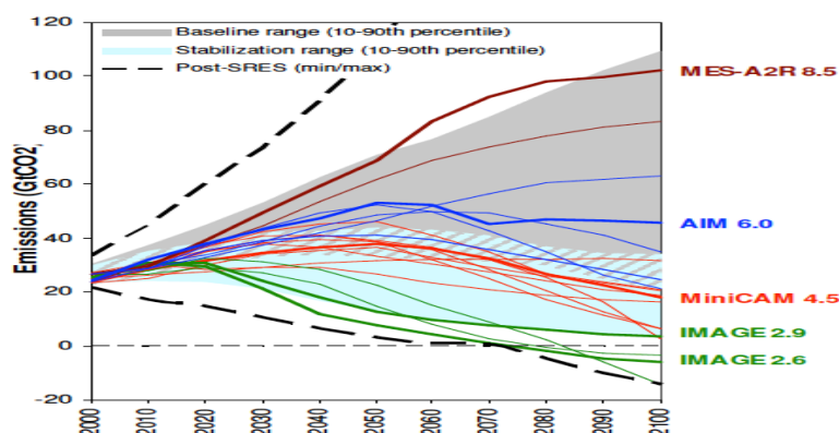
Fig.3. Evolution des émissions de CO 2 dans les scénarios du GIEC
