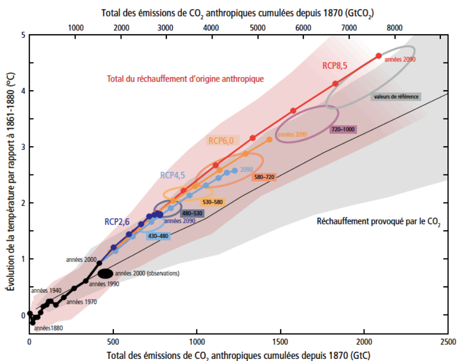
Fig.6. Réchauffement en fonction du cumul des émissions de CO 2
