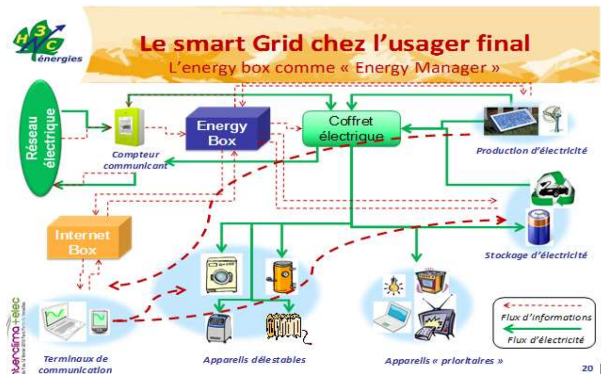
Fig. 14 : La maison intelligente avec son « energy box » - source : H3C-Energies
