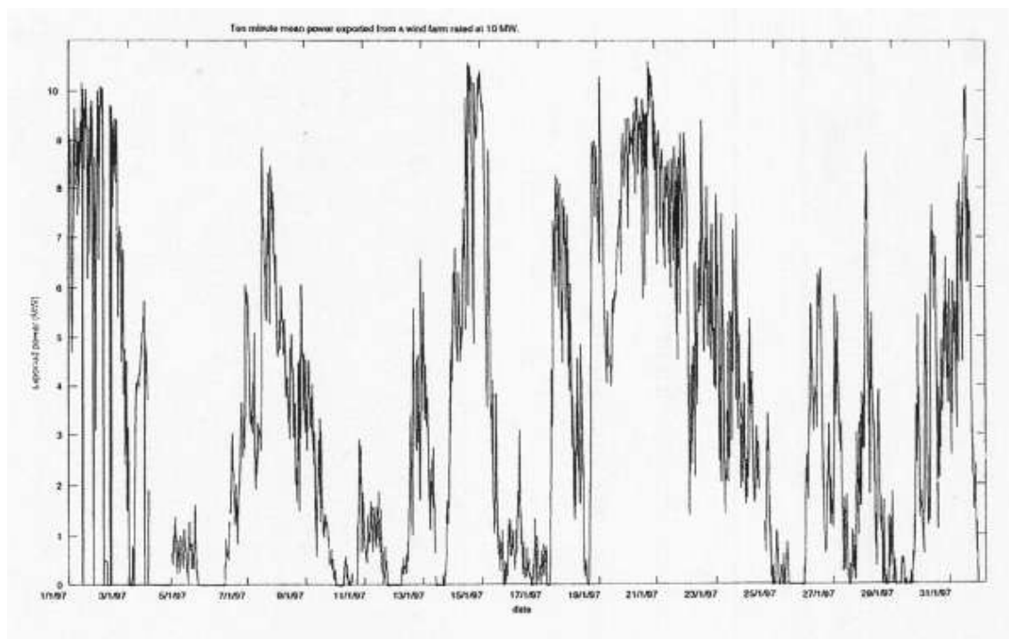
Fig. 3 : Puissance de sortie d'une ferme éolienne sur un mois (Royaume Uni)
