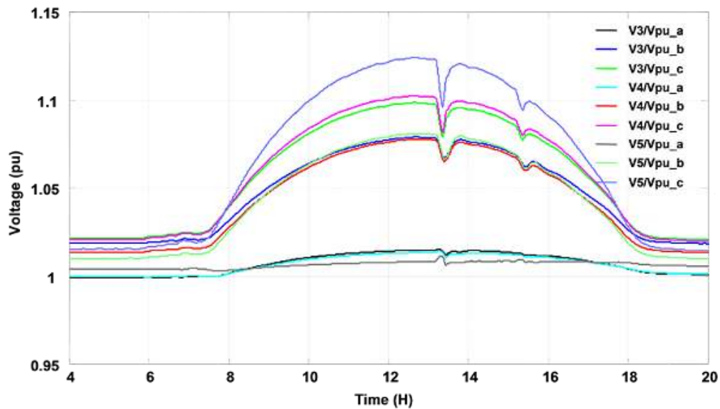
Fig. 10 : Pilotage de la tension à travers un réglage classique (Actif/Réactif ou P/Q) sur un réseau test
