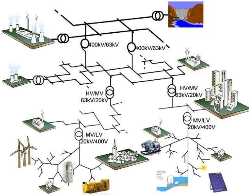
Fig. 1 : Organisation du système électrique
