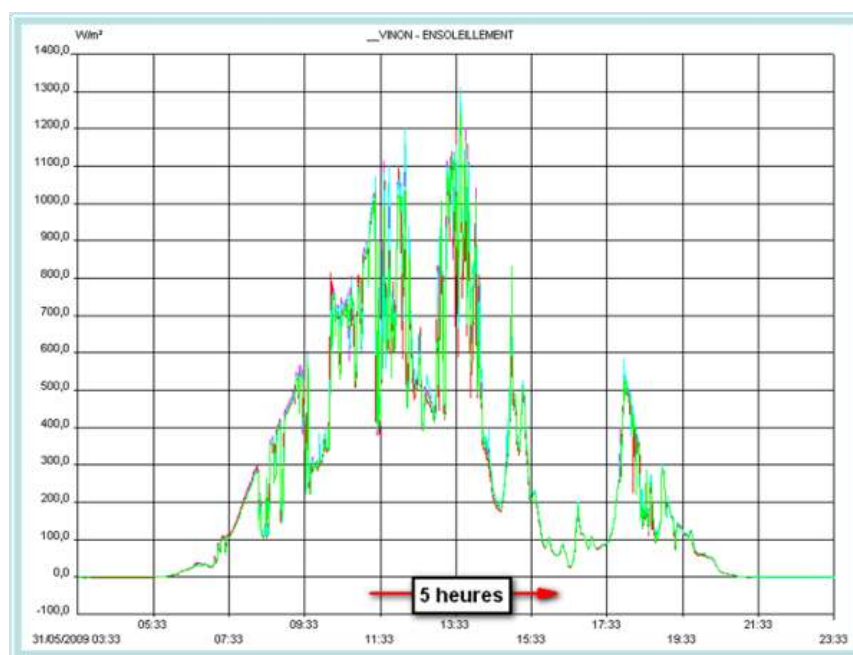
Fig. 4 : Puissance de sortie d'une ferme PV à Vinon sur Verdon (France 31 mai 2009)
