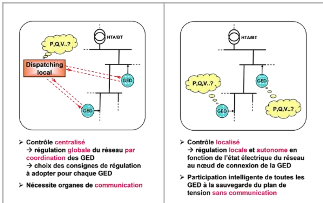
Fig. 9 : Mode de pilotage intelligent de la tension dans les réseaux de distribution en présence de production décentralisée
