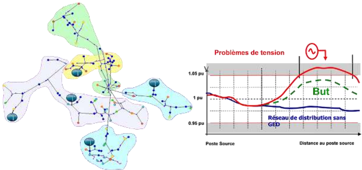
Fig. 8 : Production décentralisée et profil de tension dans les réseaux de distribution
