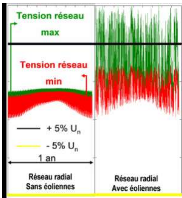
Fig. 2 : Impact du raccordement de productions éoliennes sur la tension des réseaux de distribution
