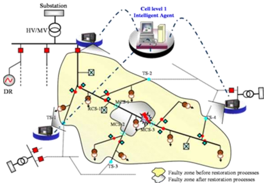
Fig. 12 : Concept du réseau auto-cicatrisant : Détecter-localiser-réparer et ré-alimenter le réseau après un défaut
