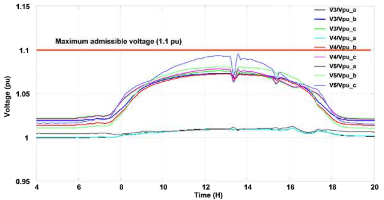
Fig. 11 : Pilotage de la tension intelligent sur un réseau test
